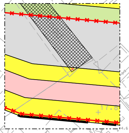
插圖D INSET D 比例 1 : 500 Scale
